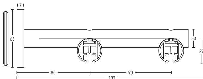
Wandträger Profil Art.-Nr. 11672-170 + 11672-190 + 11672-220
