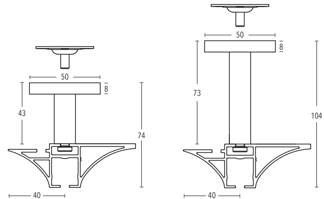
Deckenträger 43 mm + 73 mm Art.-Nr. 11473-50 + 11473-80
