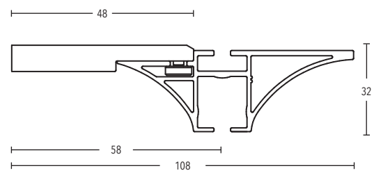
Deckenträger 5 mm Art.-Nr. 11220-20
