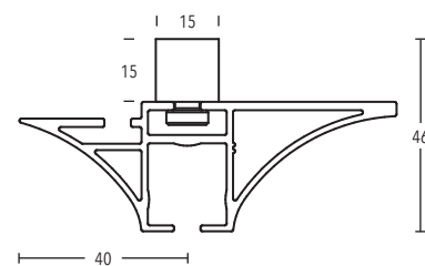
Deckenträger 15 mm Art.-Nr. 11473-100
