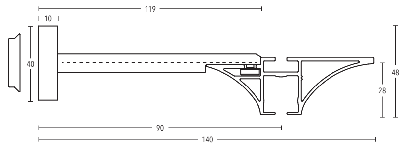
Wandträger Art.-Nr. 11220-130
