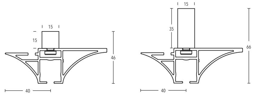
Deckenträger 15 mm + 35 mm Art.-Nr. 11473-15 + 11473-35
